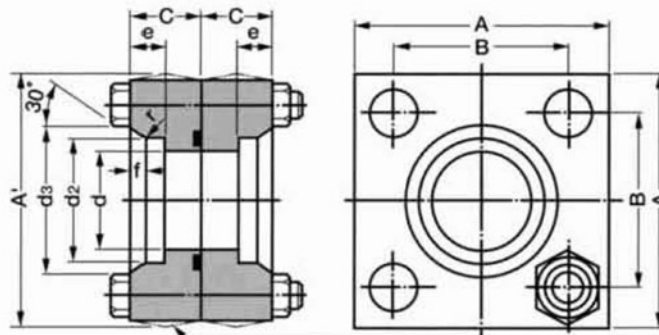
鍛造による場合の形状 Configuration by forging
